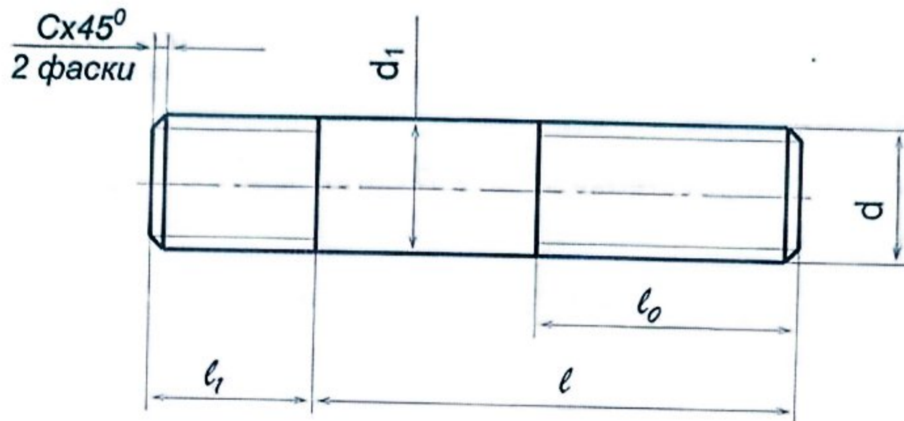
Размеры шпилек, мм
